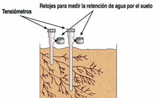
Figura 7. Tensiómetros colocados a dos profundidades distintas
