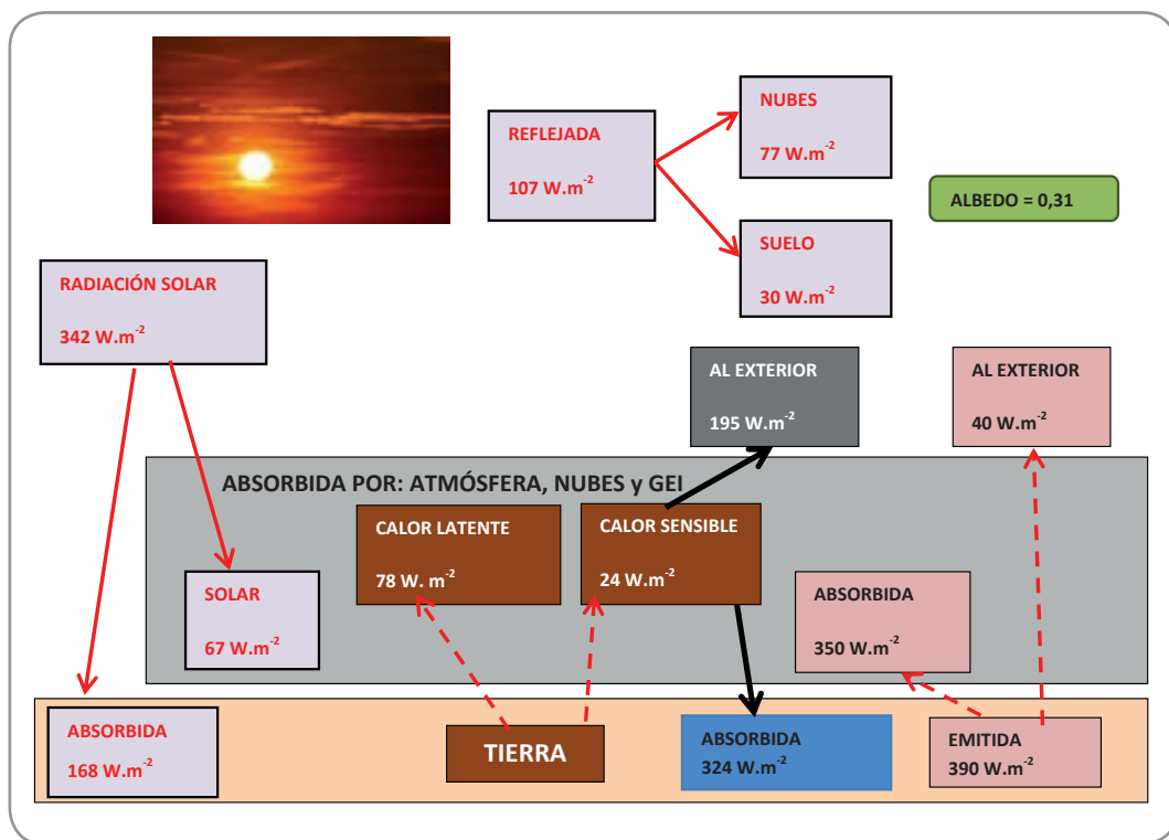
Figura 1 - Esquema del calentamiento atmosférico.
