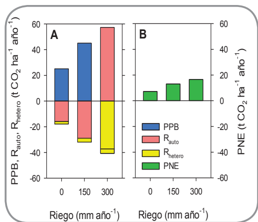
Figura 1: Valores promedio de Productividad Primaria Bruta (PPB), Respiración de los árboles (R auto ), Respiración de los organismos del suelo (Rhetero) (A), así como de su resultante, la Productividad Neta del Ecosistema (PNE) (B) para la plantación de olivar en seto simulada bajo tres escenarios de uso del agua. Valores positivos indican flujo de carbono desde la atmósfera a la plantación.
