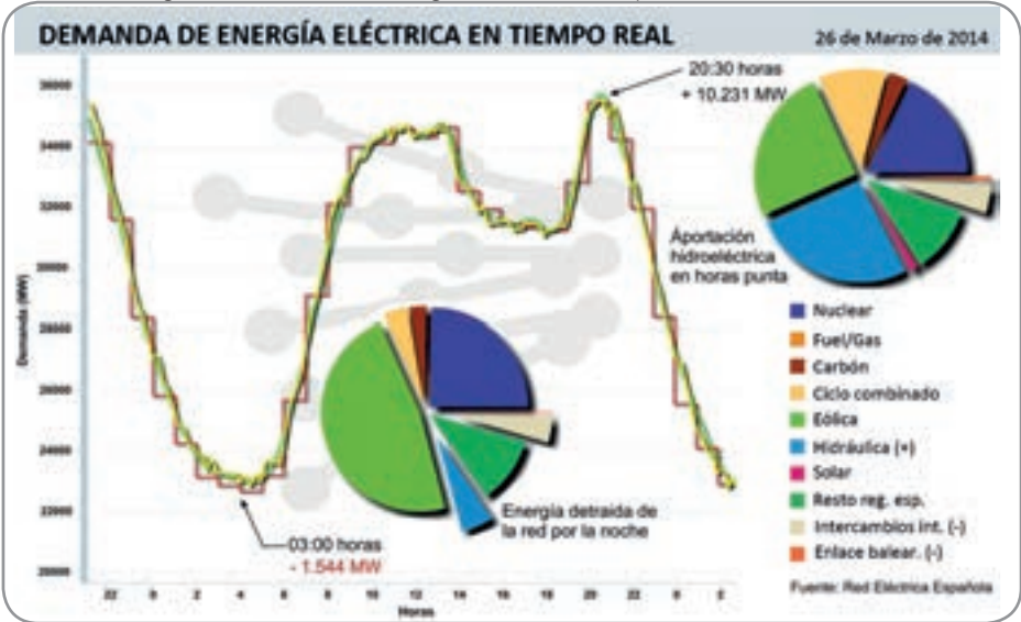
Figura 2: Demanda de energía eléctrica en tiempo real (26/03/2014).
