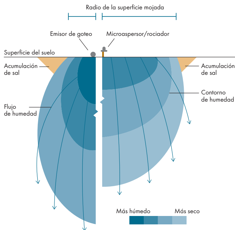
Figura 7. Patrones de humectación de la irrigación por goteo y microaspersión
