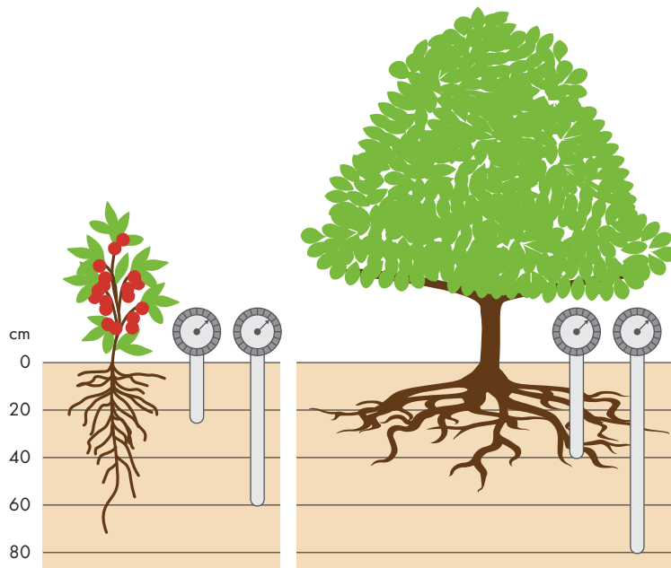
Normalmente, las sondas se colocan en 25 cm y 60 cm profundidad del suelo para los cultivos anuales, y en 40 cm y 80 cm para los cultivos perennes y los cultivos de árboles.
