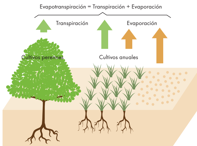
Figura 4. Evapotranspiración
