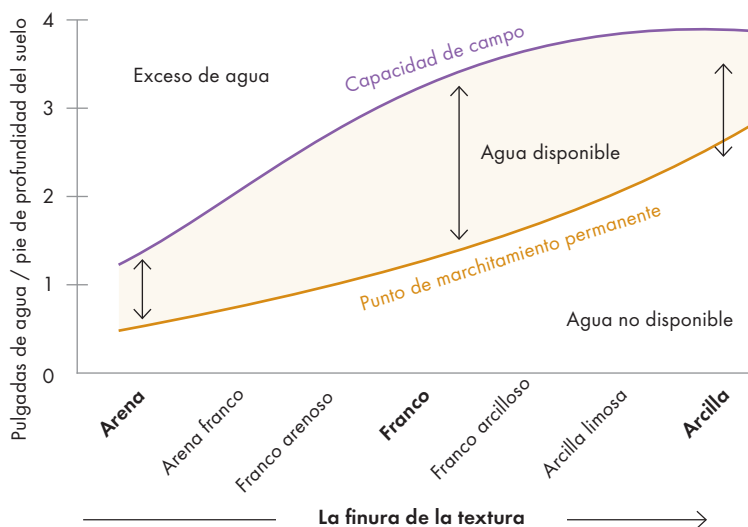
Figura 2. Relación entre la capacidad de campo y el agua disponible en diferentes tipos de suelo
