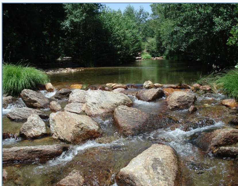
Foto 21. Rampa para el paso de peces en el río Negro (Zamora) ejecutada por la Confederación Hidrográfica del Duero.
